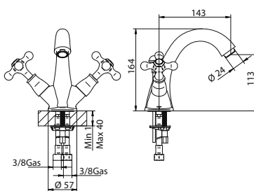
Monoforo lavabo Washbasin tap mixer Waschtischbatterie Monoforo lavabo Monotrou de lavabo
